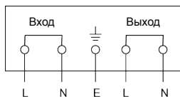
Рис. 9. Принципиальная схема проводки изделий ТМ-3 – ТМ-10
