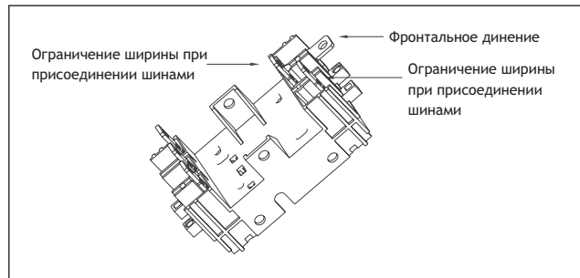
Втычное исполнение
