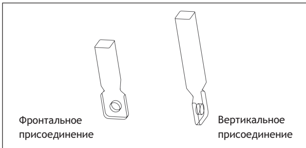
Присоединение шинами
