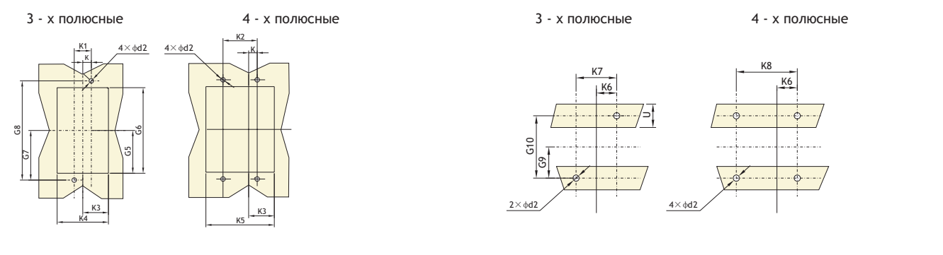
Разметка монтажной панели
