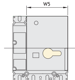
4 - х полюсный
