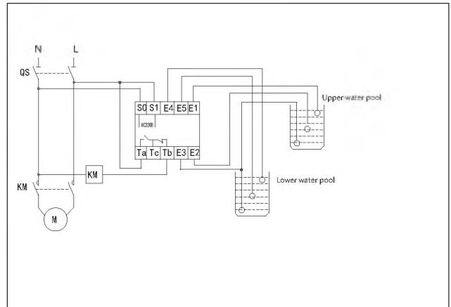
Для NYW1-BL1, NYW1-BL2 напряжение питания 220V
