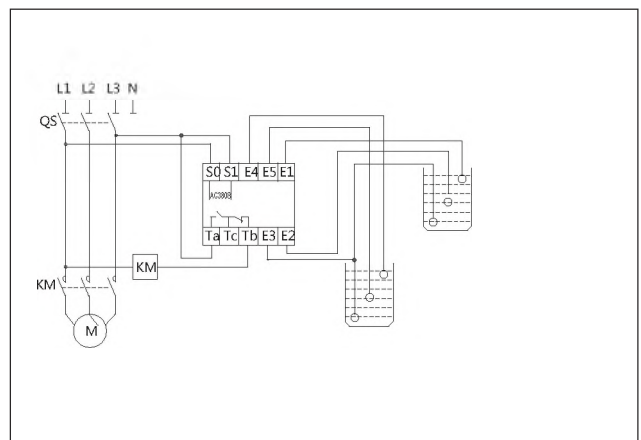
Для NYW1-BL1, NYW1-BL2 напряжение питания 380V
