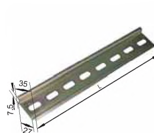
Размеры монтажной рейки
