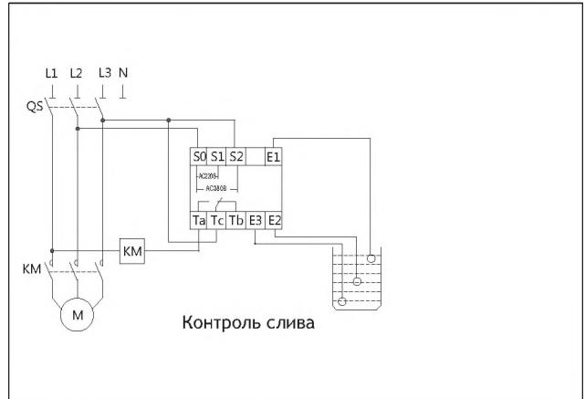
Для NYW1-NL1, NYW1-NL2 напряжение питания 220V/380V
