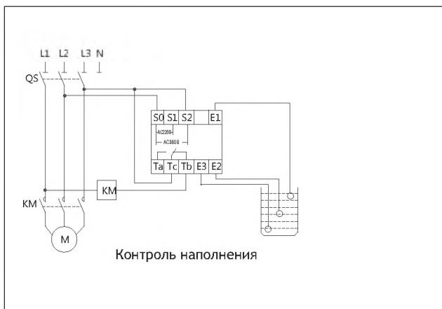
Для NYW1-NL1, NYW1-NL2 напряжение питания 220/380V
